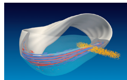
核融合科学研究所 プラズマの粒子シミュレーション
